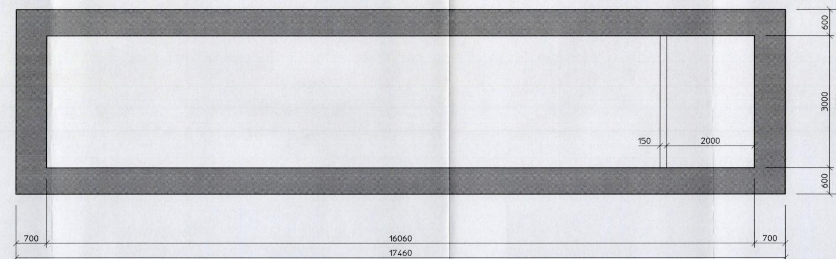
Doorsnede I
