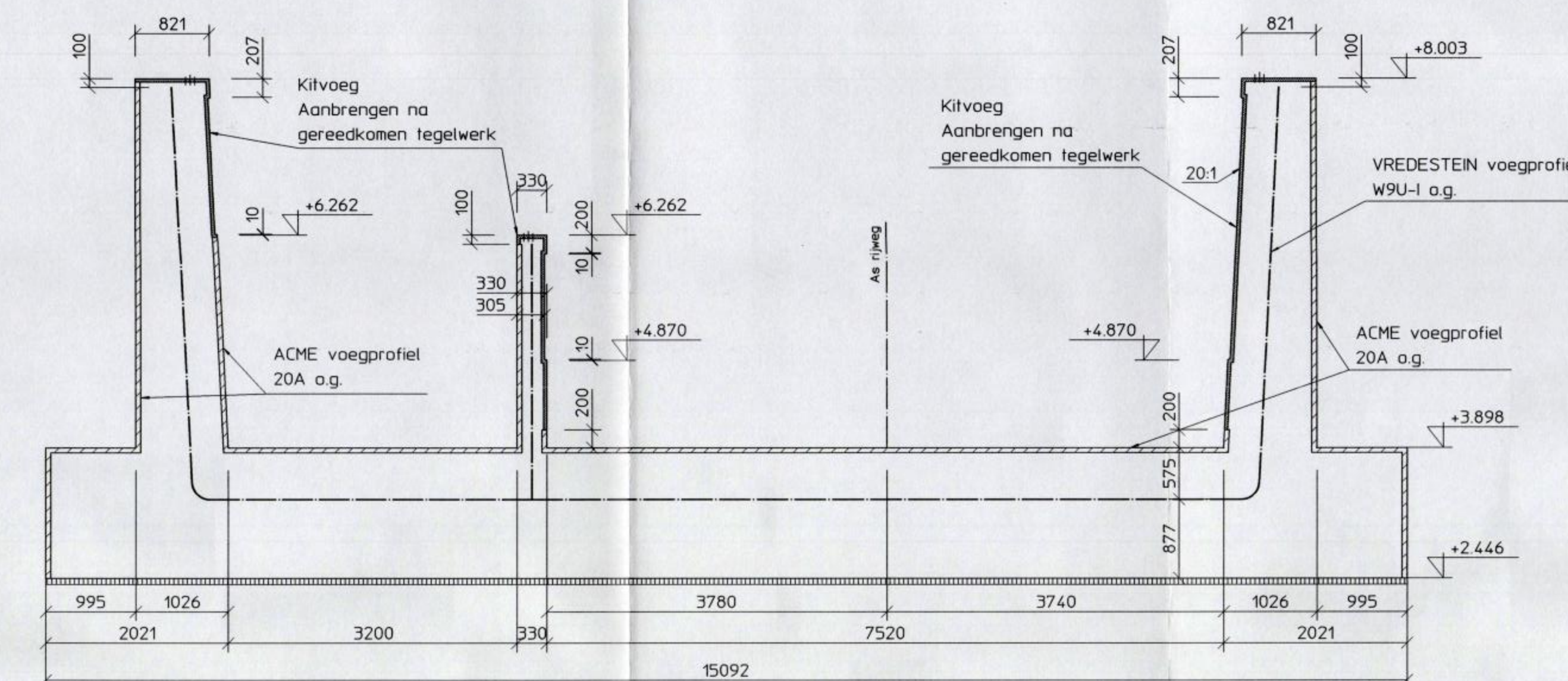
Aanzicht G
