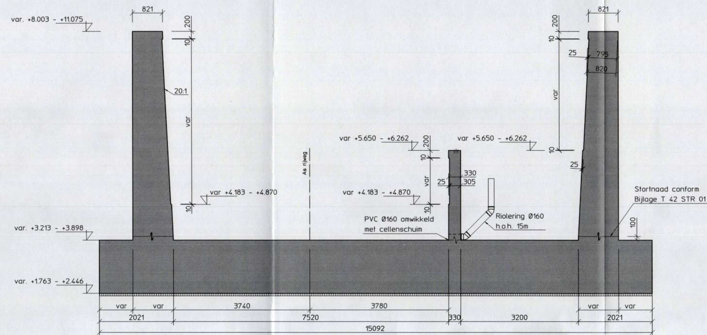
Doorsnede D
