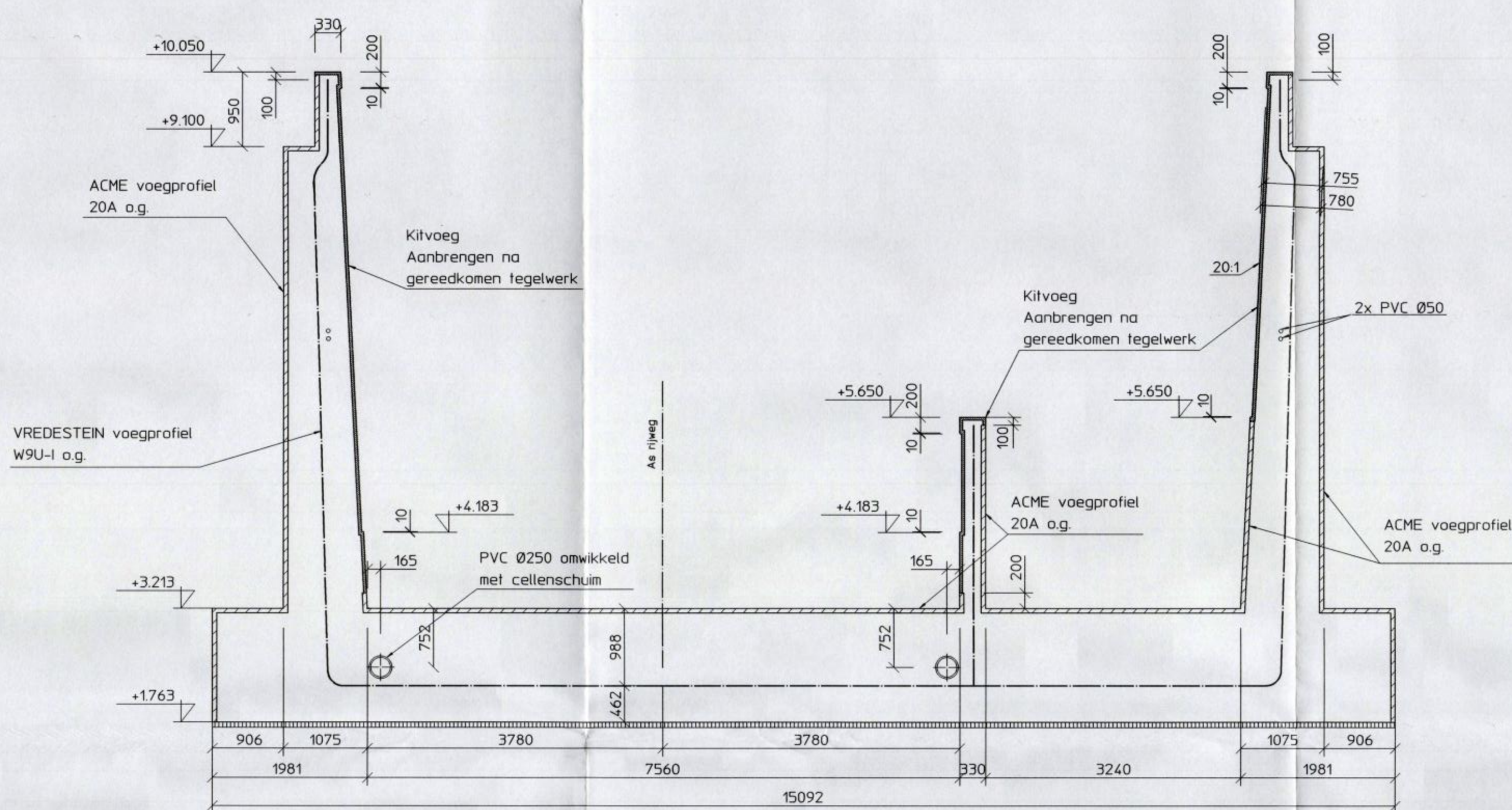
Aanzicht F
