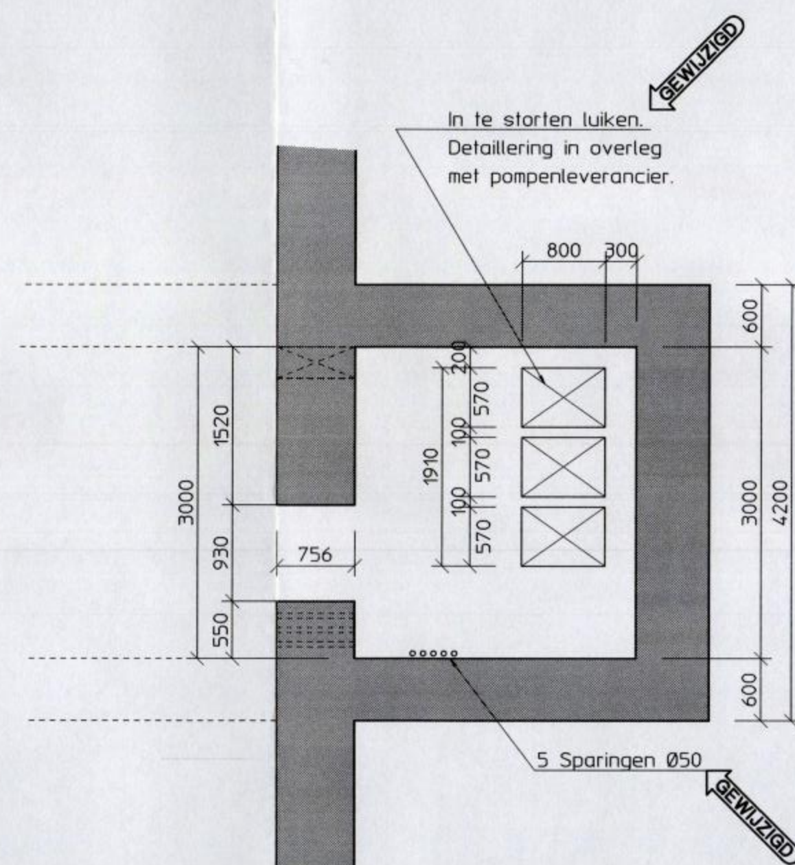
Doorsnede H
